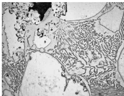
6. kép: Dombóvár, Gólyavár. Bronz ágyú töredékének öntött, lassan hűlő alapanyagra utaló csiszolati képe
